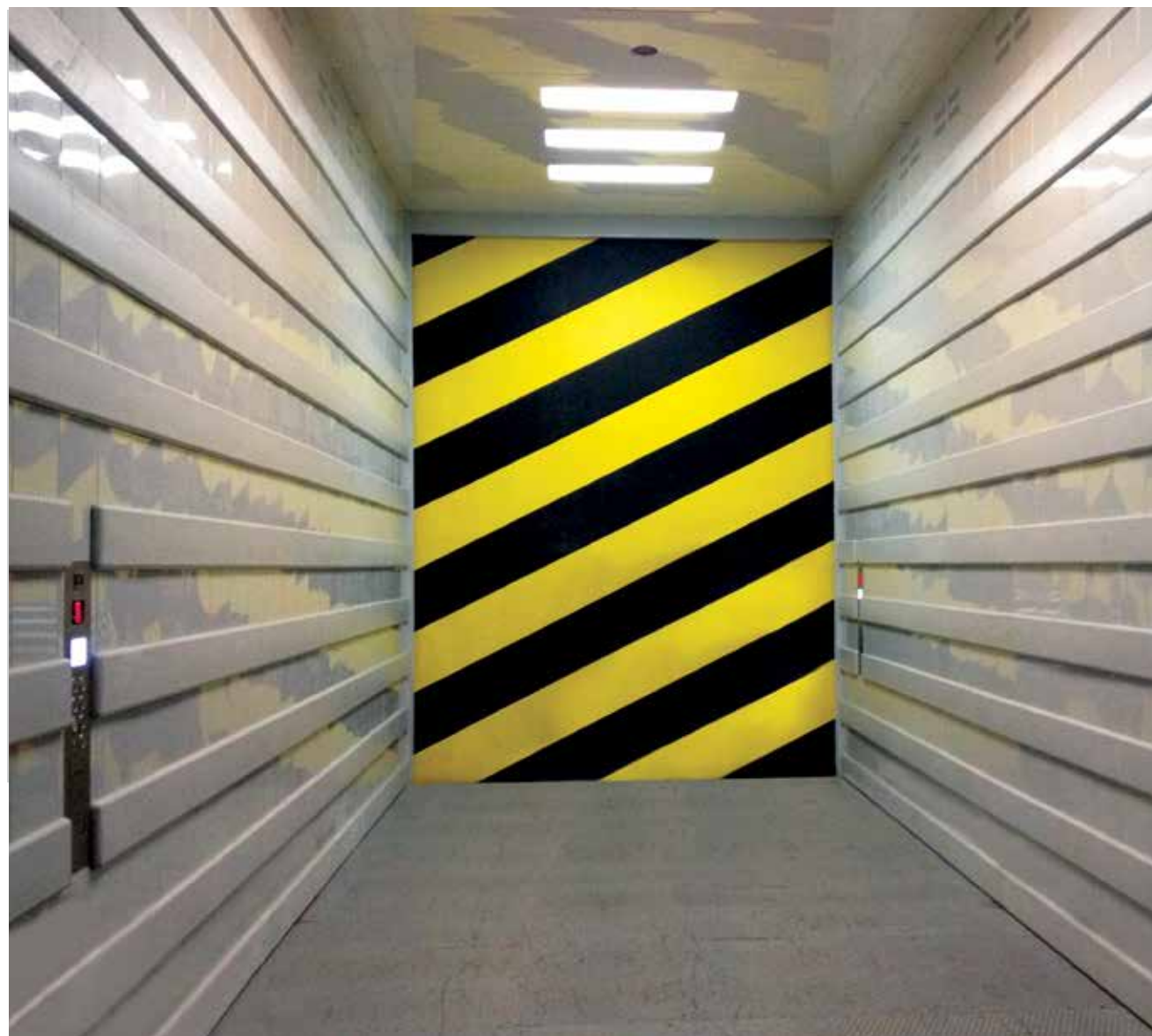
Custom-made Hydraulic Freight Lift 3,6 m wide x 8m depth x 4,7 m height Kundenspezifischer Hydraulikaufzug 3,6m Breite x 8m Tiefe x 4,7 Höhe
